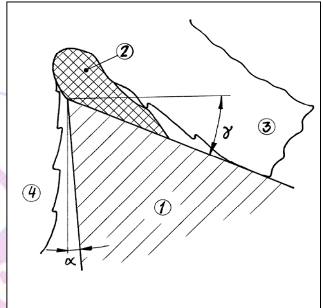
figuur 1: Vorming van een valse snijkant. 1. beitel, 2. valse snijkant, 3. spaan, 4. oppervlaktegesteldheid, \alpha vrijloophoek, \gamma spaanhoek
