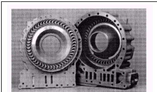
Figuur 5 Hard geanodiseerd gietwerk
