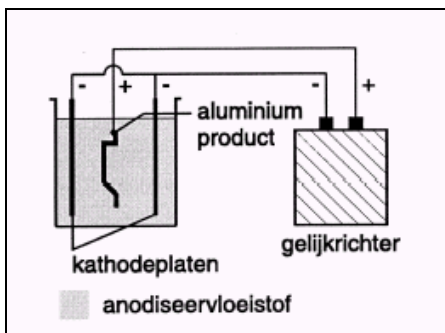
Figuur 1 Principe van anodiseren
