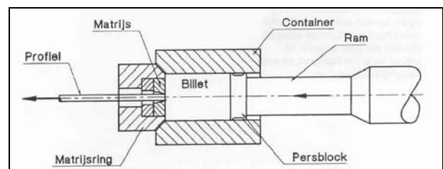
figuur 2: schematische voorstelling van het extrusieproces.
