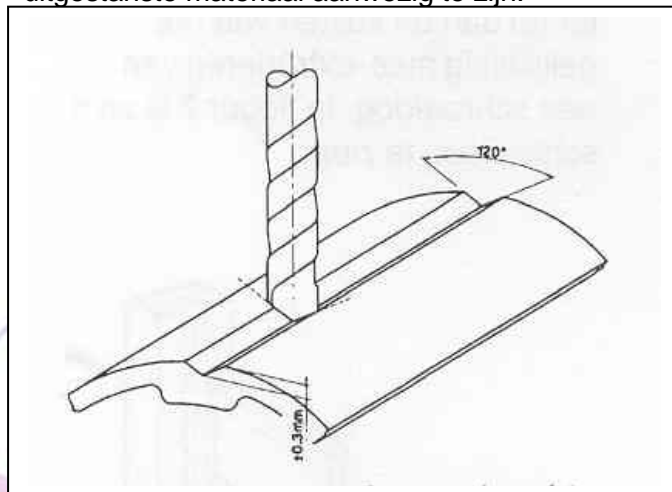
figuur 9: geïntegreerde functie voor mechanische nabewerking.
