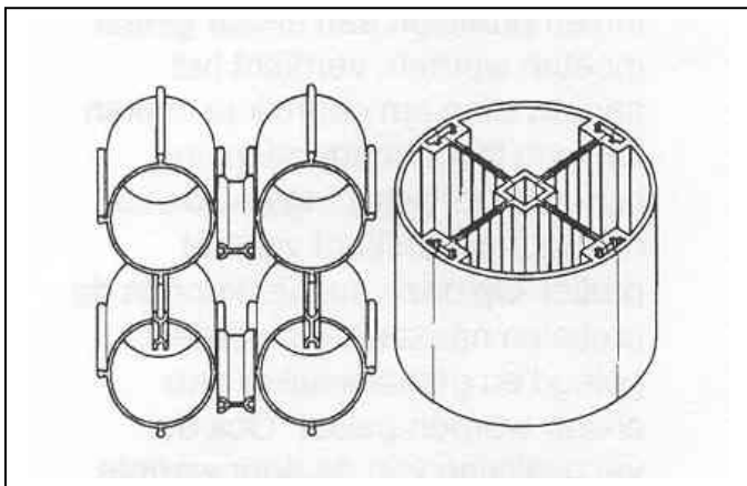
figuur 7: samengestelde extrusieprofielen
