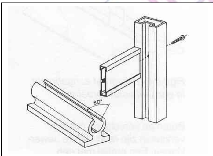
figuur 8: montage voordelen door integreren van schroefoog.
