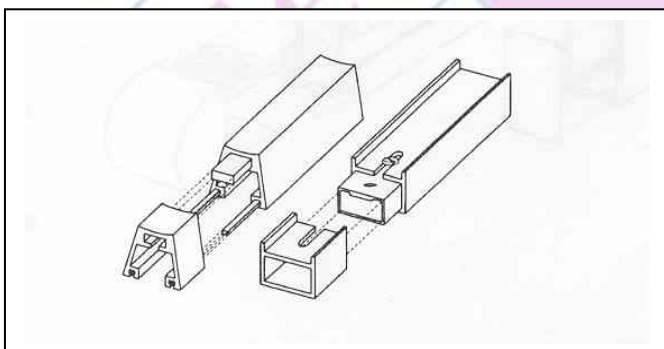
figuur 4: samenvoegen van profielen tot één geheel.
