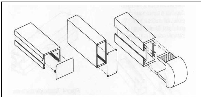
figuur 3: eindafsluitingen.
