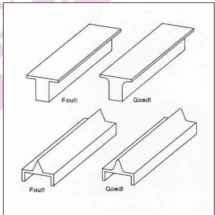
figuur 13: constructieaanbevelingen.
