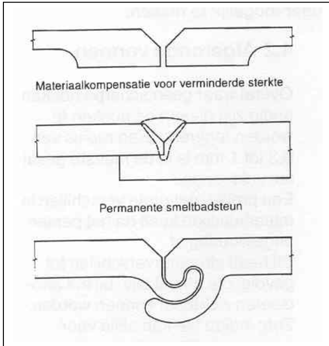
figuur 11: voorbeelden van meegeëxtrudeerde lasbadondersteuning.
