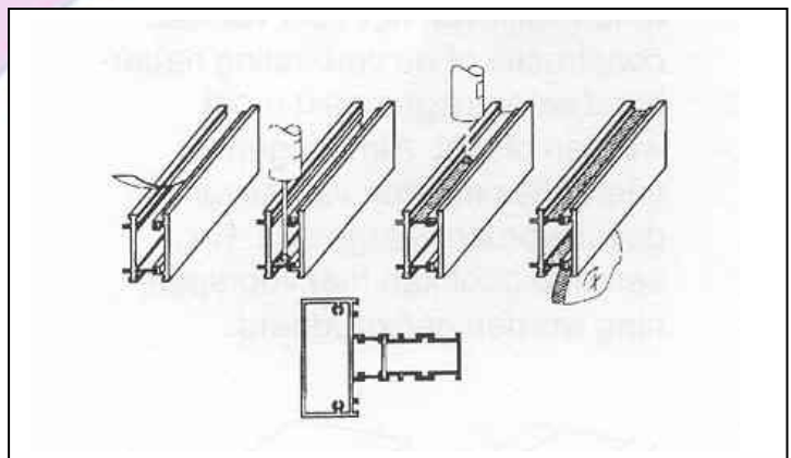
figuur 6: door toepassing van kunststof is een koudebrug zorg dragen voor isolatie.
